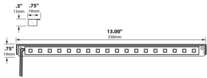
SL-43LG-LEDs
