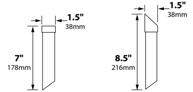
SL-36-MR8
