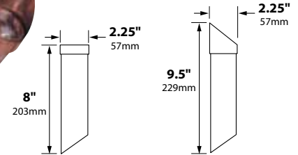
SL-36-MR16
