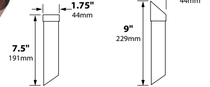
SL-36-MR11
